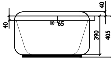
END ELEVATION
