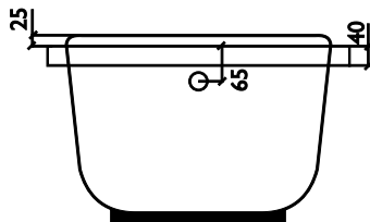
END ELEVATION
